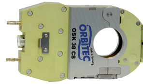
Geschlossene Schweißzange OSK 38 CS
