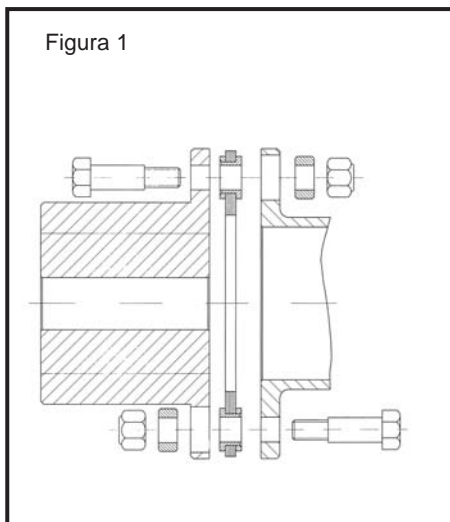
Figura 1 = Schema di montaggio pacco lamellare
