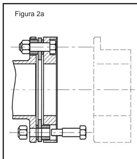
Figura 2 = Schema di montaggio pacco lamellare
