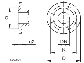
Flansche EN 1092-2
