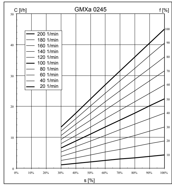
Abb. 3: Dosierleistung C bei mittlerem Gegendruck in Abhängigkeit von der Hublänge s für unterschiedliche Hubfrequenzen f
