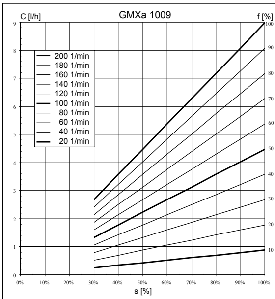
Abb. 2: Dosierleistung C bei mittlerem Gegendruck in Abhängigkeit von der Hublänge s für unterschiedliche Hubfrequenzen f
