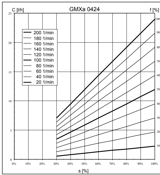
Abb. 3: Dosierleistung C bei mittlerem Gegendruck in Abhängigkeit von der Hublänge s für unterschiedliche Hubfrequenzen f
