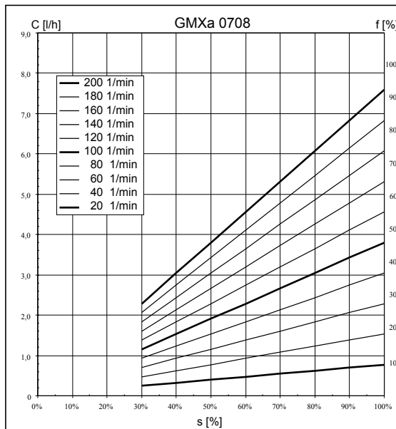
Abb. 1: Dosierleistung C bei mittlerem Gegendruck in Abhängigkeit von der Hublänge s für unterschiedliche Hubfrequenzen f
