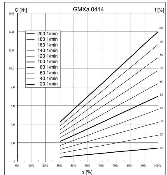
Abb. 1: Dosierleistung C bei mittlerem Gegendruck in Abhängigkeit von der Hublänge s für unterschiedliche Hubfrequenzen f
