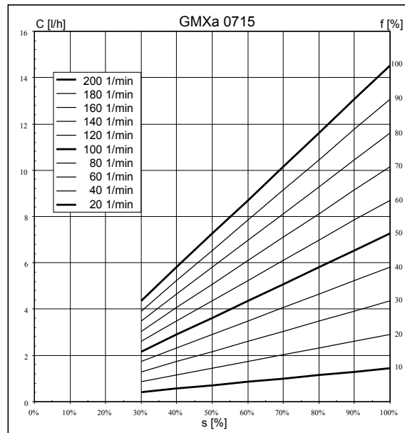
Abb. 2: Dosierleistung C bei mittlerem Gegendruck in Abhängigkeit von der Hublänge s für unterschiedliche Hubfrequenzen f
