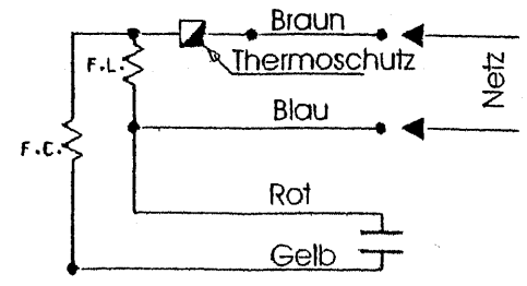
Anschlußschema
